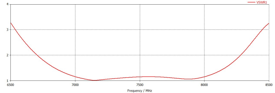
График КСВ в рабочем диапазоне частот
