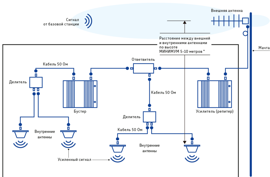
Рис. 3 Пример разветвленной системы усиления с использованием линейного усилителя мощности
