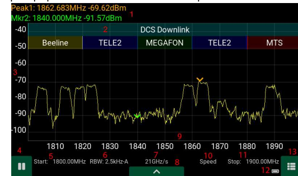
Информация на экране прибора
