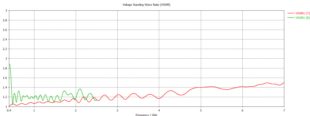
График КСВ в рабочем диапазоне
