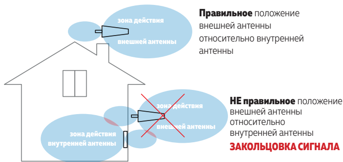
Рисунок 3 - Схема расположения внешней и внутренней антенны относительно друг друга
