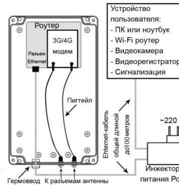
Пример размещения оборудования в гермобоксе
