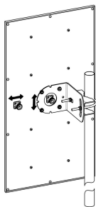
Рисунок 2 – Монтаж антенны на мачте
