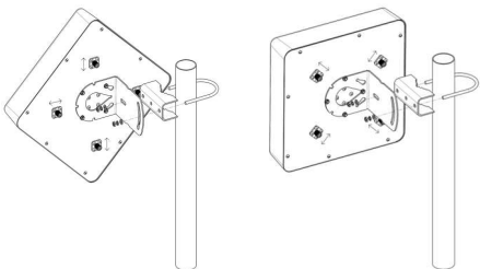
Монтаж антенны на мачте в + поляризации (слева) и в х – поляризации (справа).
