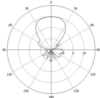
Частота 3800 МГц (0°) Усиление 9,7 дБи
