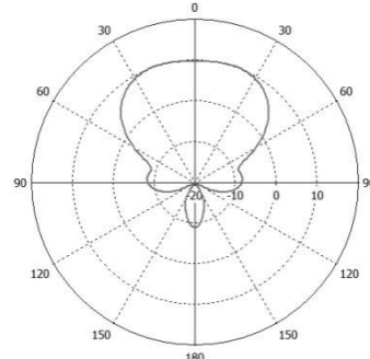
Частота 3800 МГц (90°) Усиление 9,7 дБи
