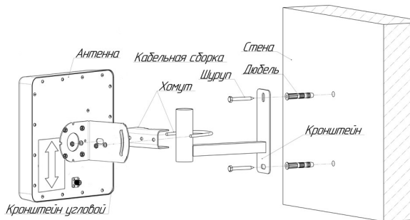
Рисунок 2 – Монтаж антенны
