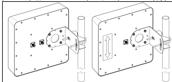
Рисунок 2 – Монтаж антенны на мачте
